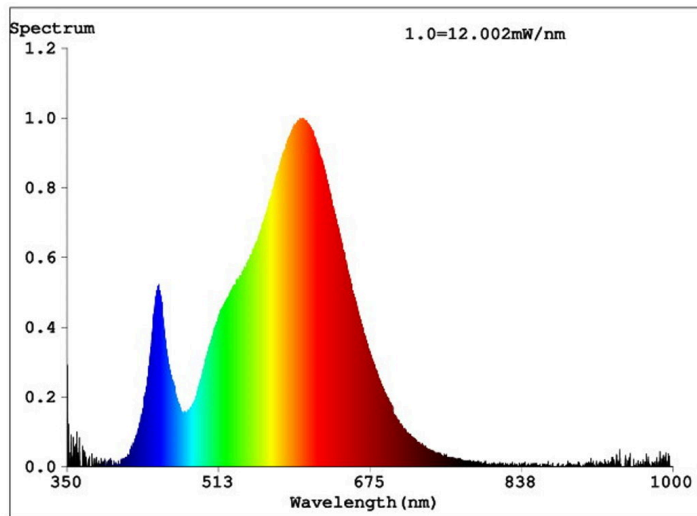
Spektrale Lichtverteilungskurve
