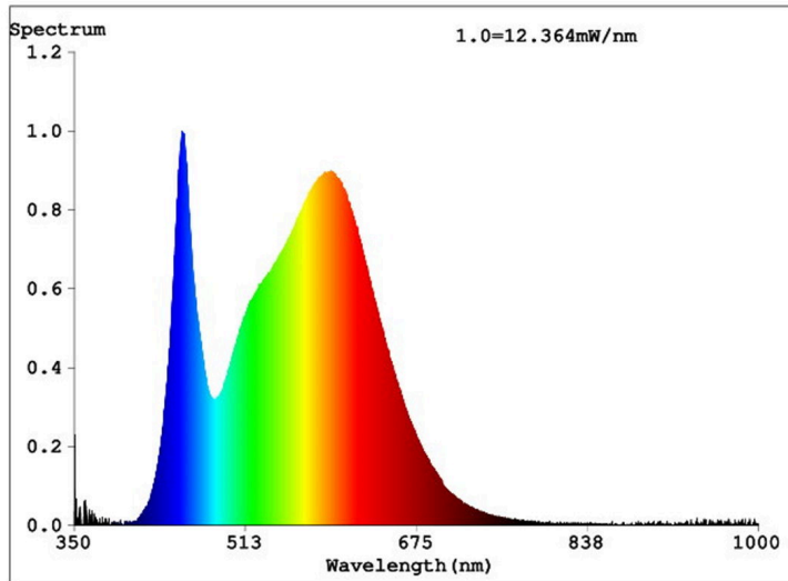
Spektrale Lichtverteilungskurve
